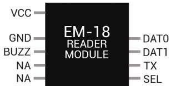
Fig. 10 EM18 Reader
